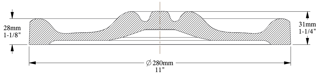
SECTION A-A SCALE 1:2
